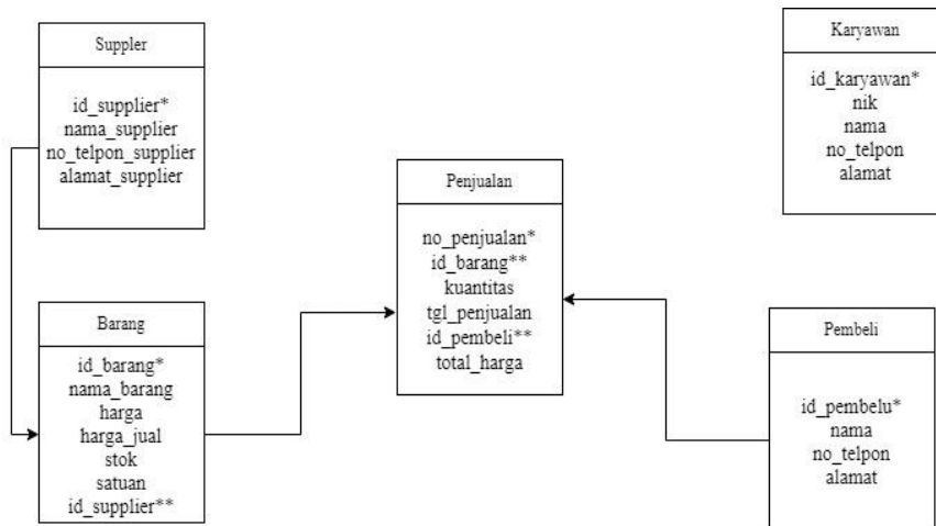
Gambar 2. Normalisasi
