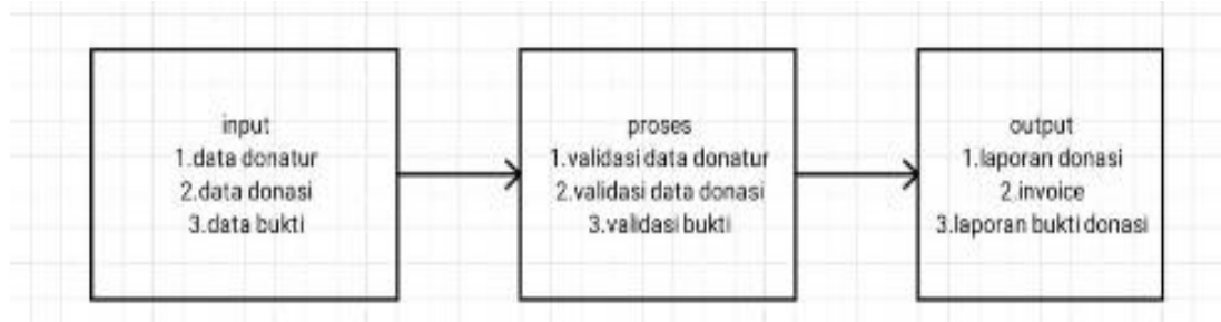
Gambar 1. Kerangka Sistem
