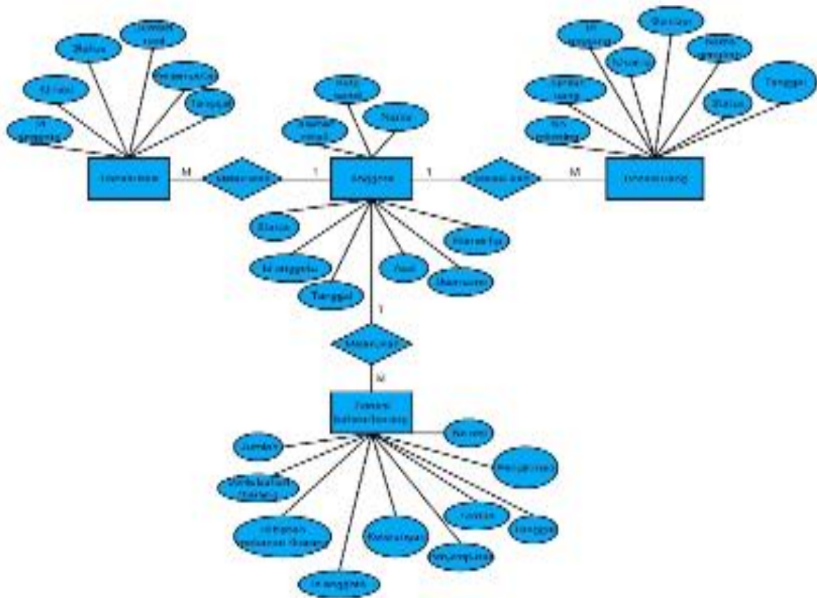
Gambar 4. ERD
